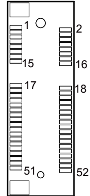
M_PCIE1
