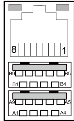
LAN1_USB1
