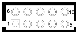
COM3/ COM4 Pin Header
