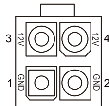
ATX_PWR2
