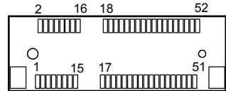
M_PCIE1
