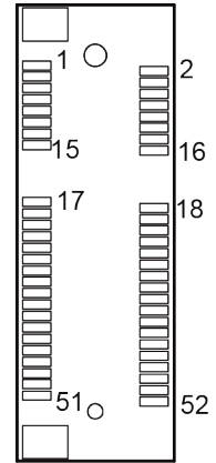
M_PCIE1
