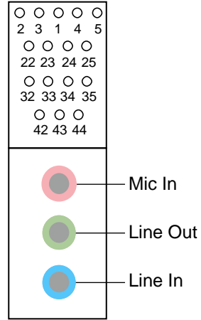
AUDIO1
