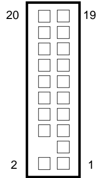
JLPC1
